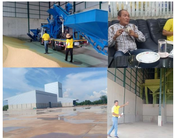
สหกรณ์การเกษตรด่านขุนทดจำกัด จ.นครราชสีมา เครื่องสีข้าวโพด ขนาด 20 ตัน/ชม. ลานตาก ขนาด 8,490 ตรม. เครื่องอบลดความชื้นพร้อมโรงคลุม 500 ตัน โกดัง 8,000 ตัน
